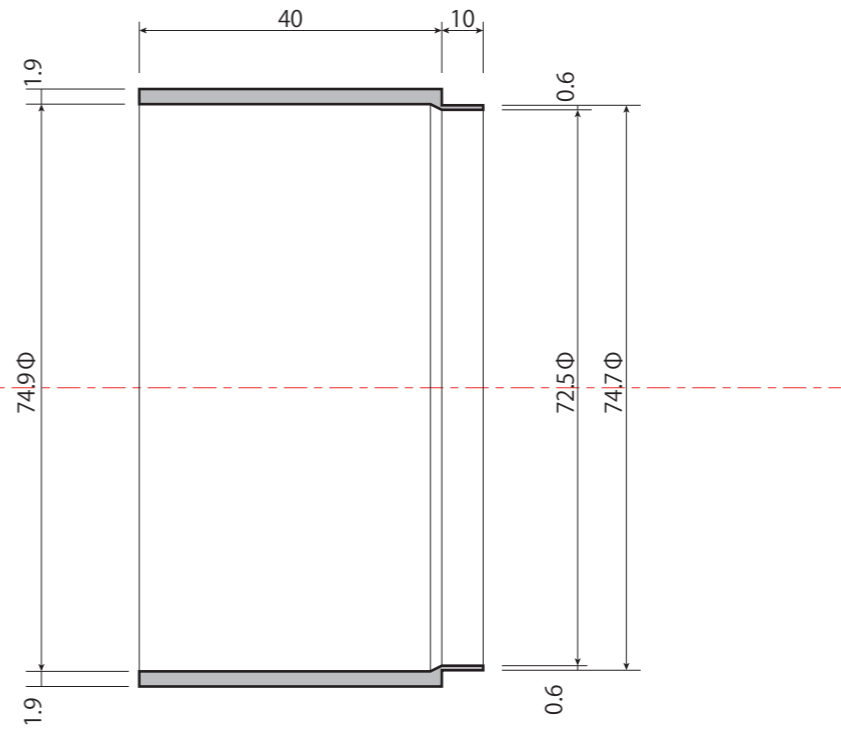
A-A 断面図
